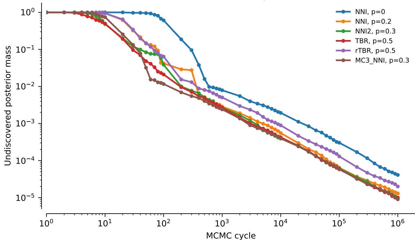
vert.coii.tw5: undiscovered posterior mass
