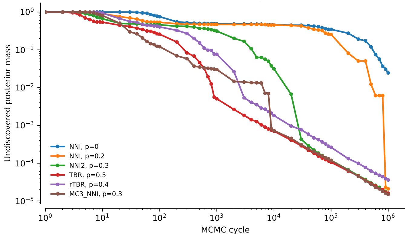
vert.coiii.tw2: undiscovered posterior mass
