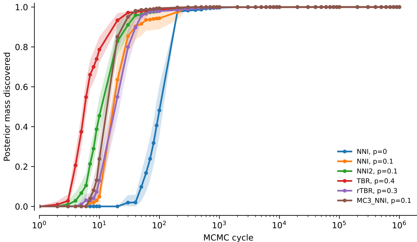
vert.nd1.tw0: Posterior mass discovered
