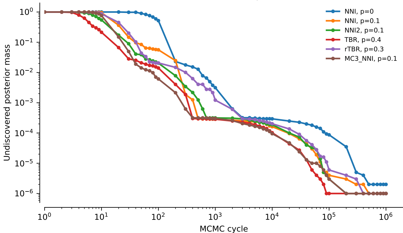
vert.nd1.tw0: undiscovered posterior mass
