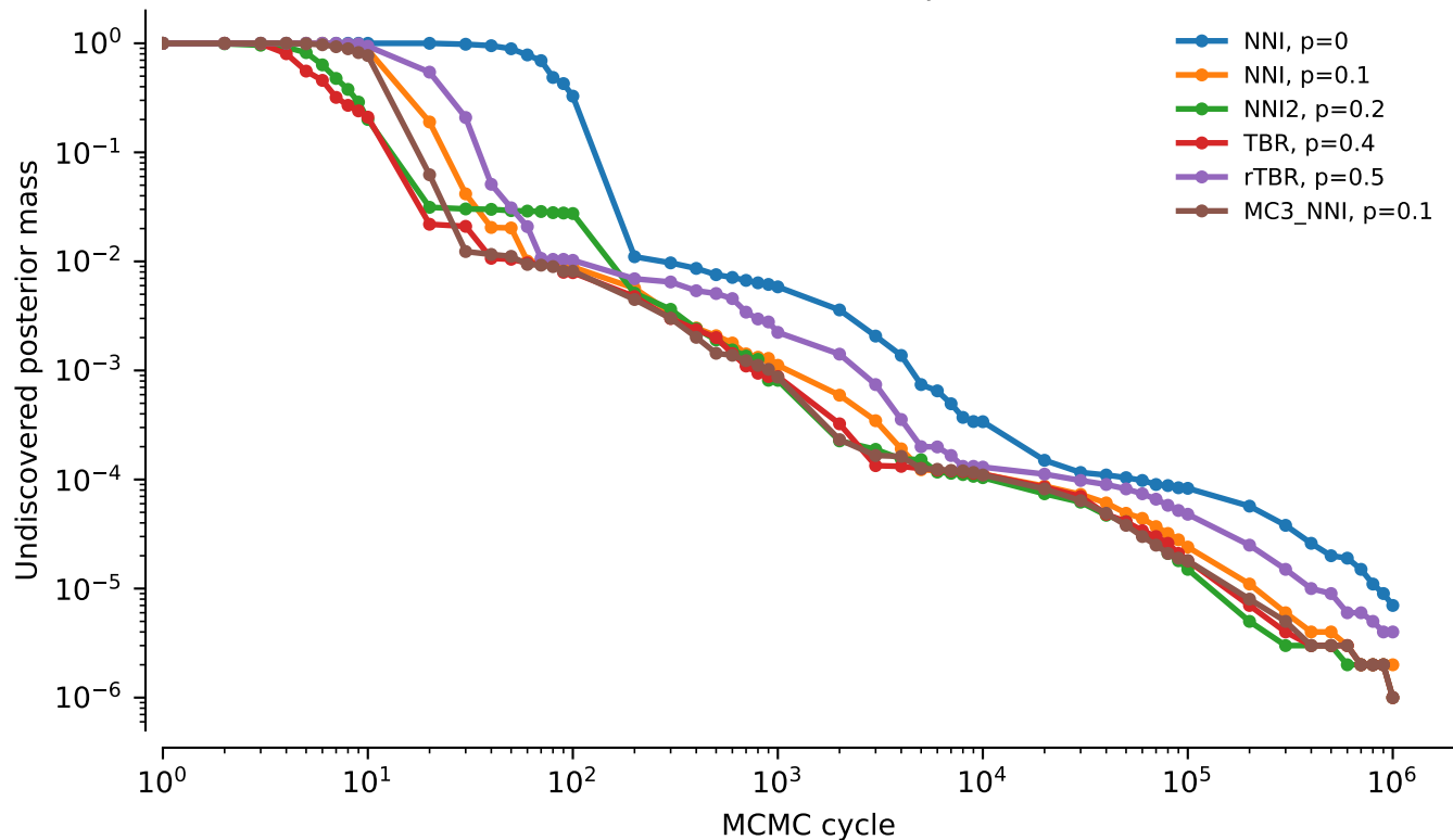
vert.nd2.tw0: undiscovered posterior mass
