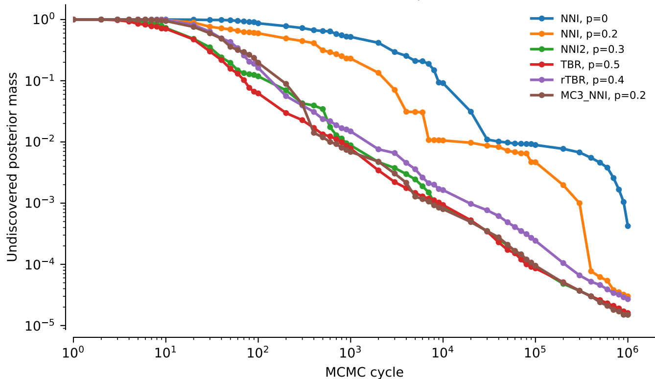
vert.nd2.tw5: undiscovered posterior mass
