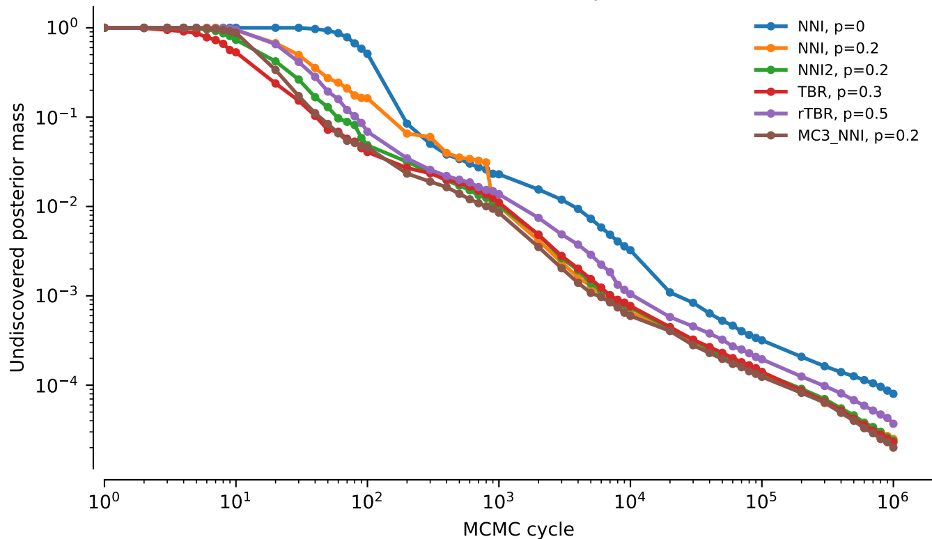
vert.nd3.tw0: undiscovered posterior mass
