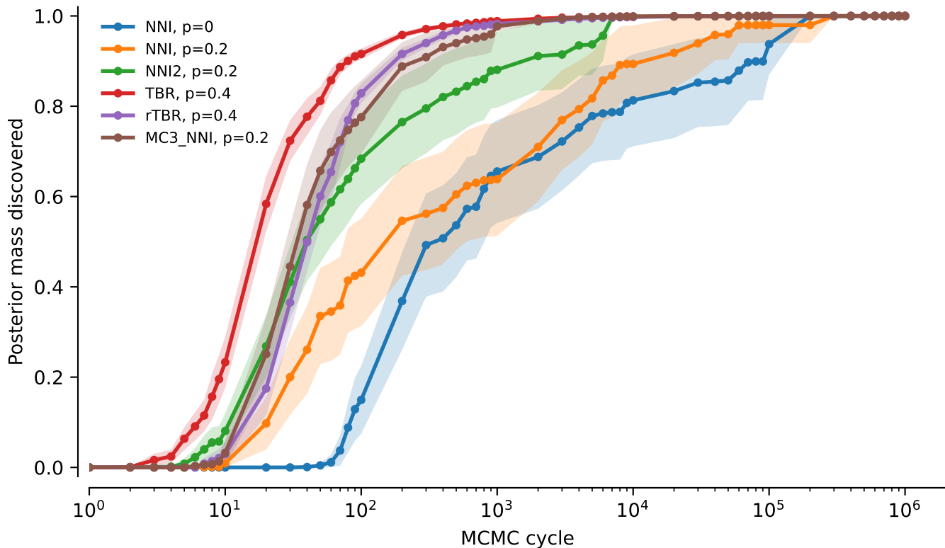
vert.nd3.tw5: Posterior mass discovered
