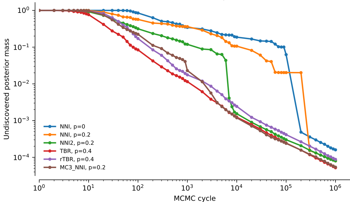
vert.nd3.tw5: undiscovered posterior mass
