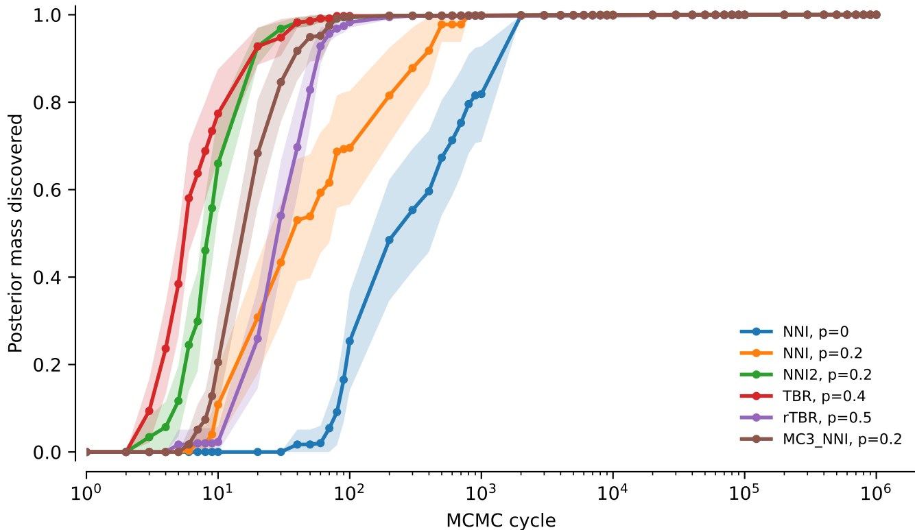
vert.nd4.tw5: Posterior mass discovered
