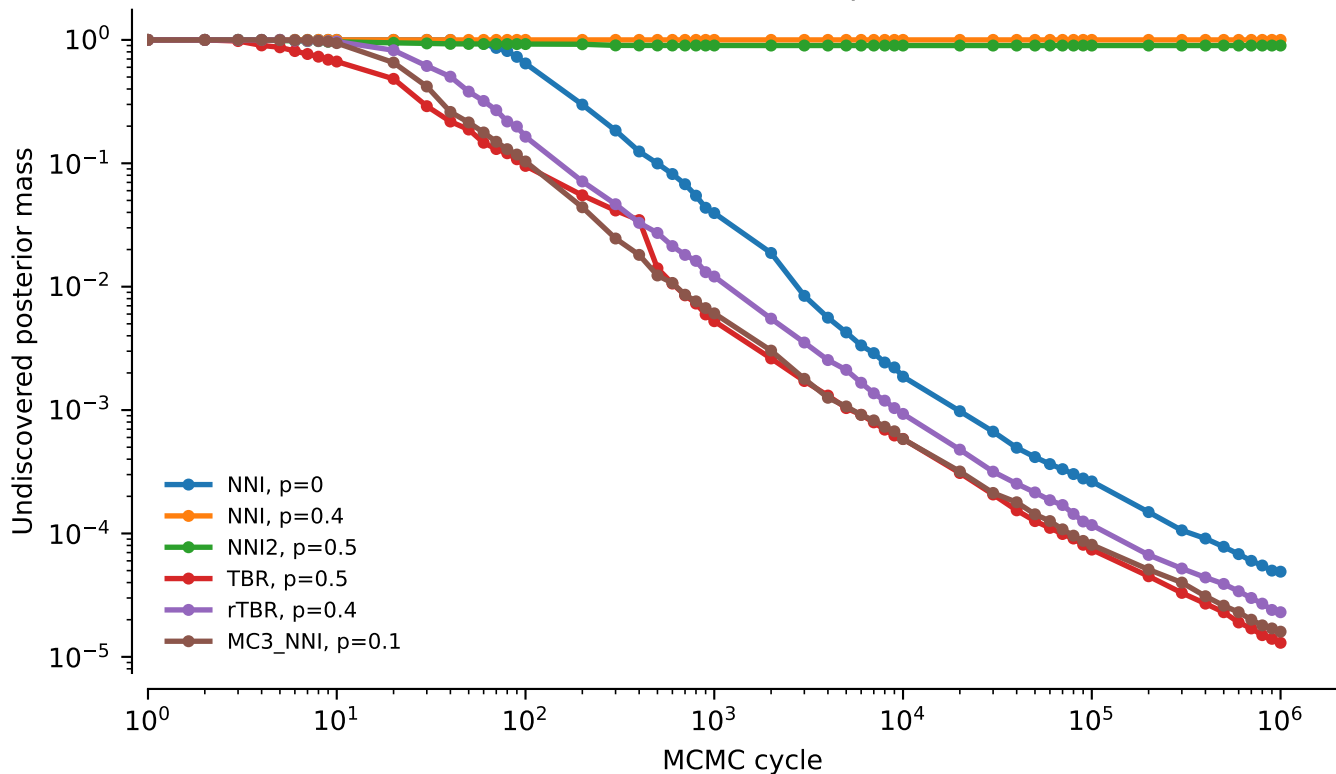
vert.nd6.tw0: undiscovered posterior mass
