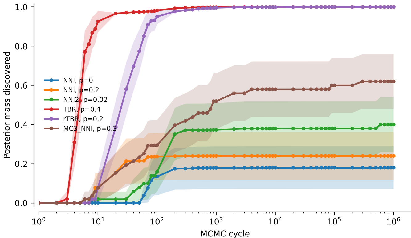
vert.nd6.tw5: Posterior mass discovered
