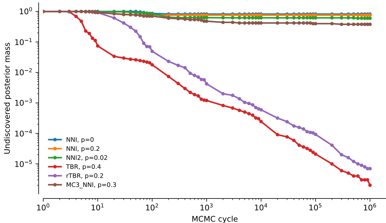
vert.nd6.tw5: undiscovered posterior mass
