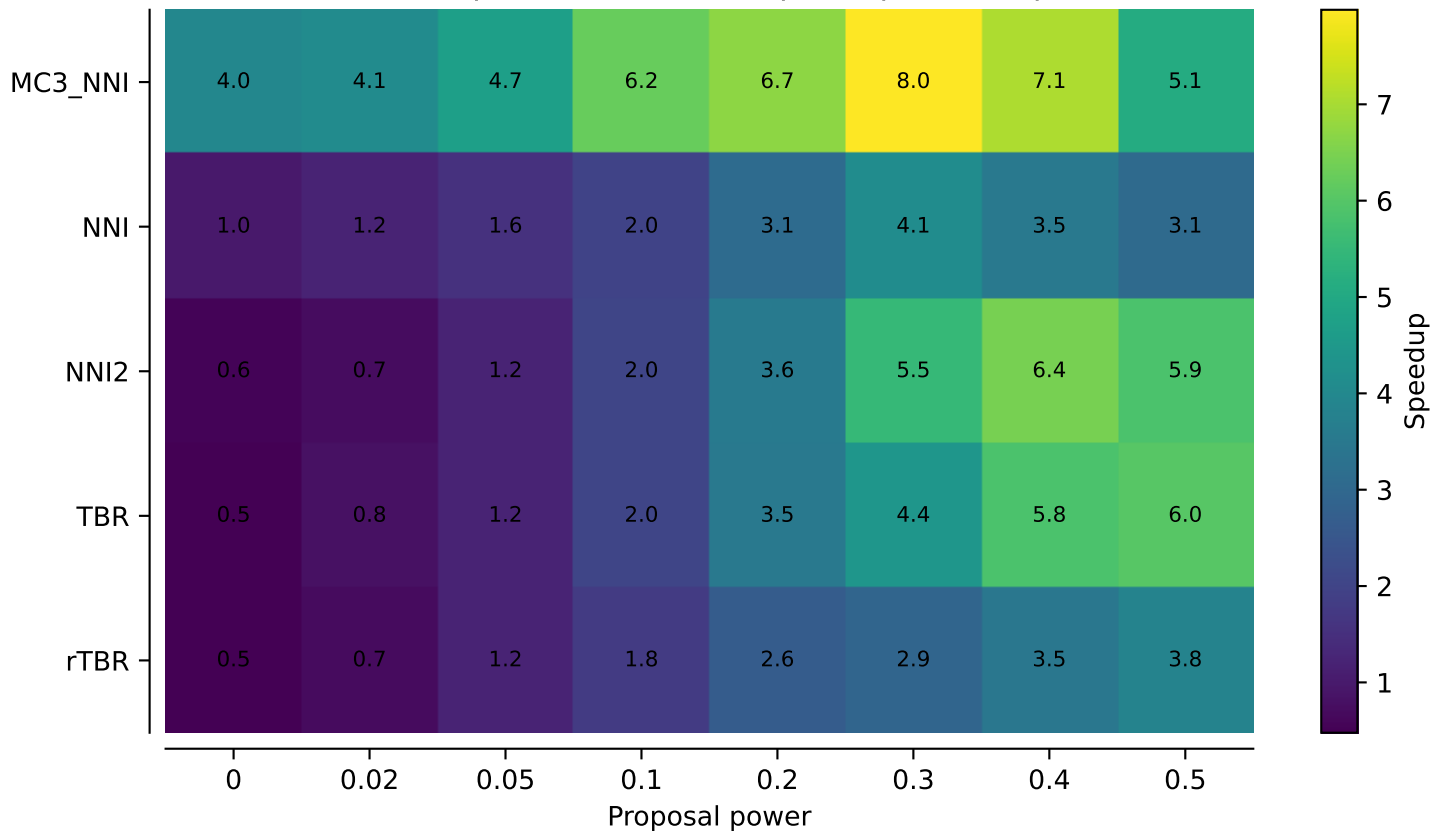
vert.atpase8.tw5: tau95 speedup heatmap
