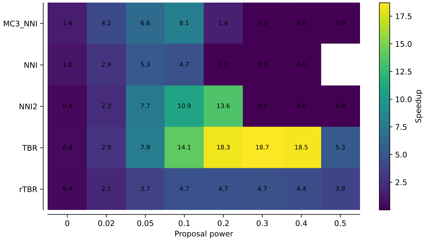
vert.nd4.tw0: tau95 speedup heatmap
