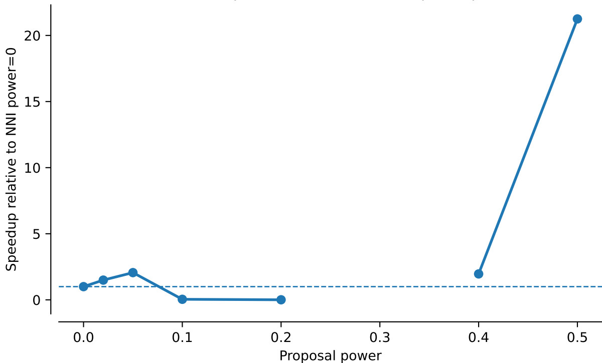
vert.atpase6.tw0: NNI tau95 speedup
