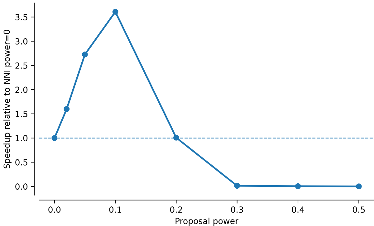
vert.atpase6.tw5: NNI tau95 speedup
