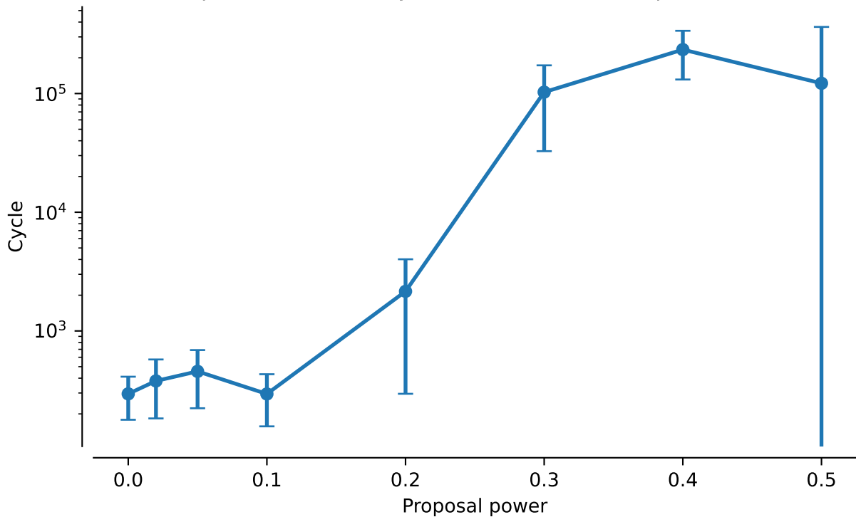
vert.atpase8.tw0: NNI Cycles to discover 95% posterior mass
