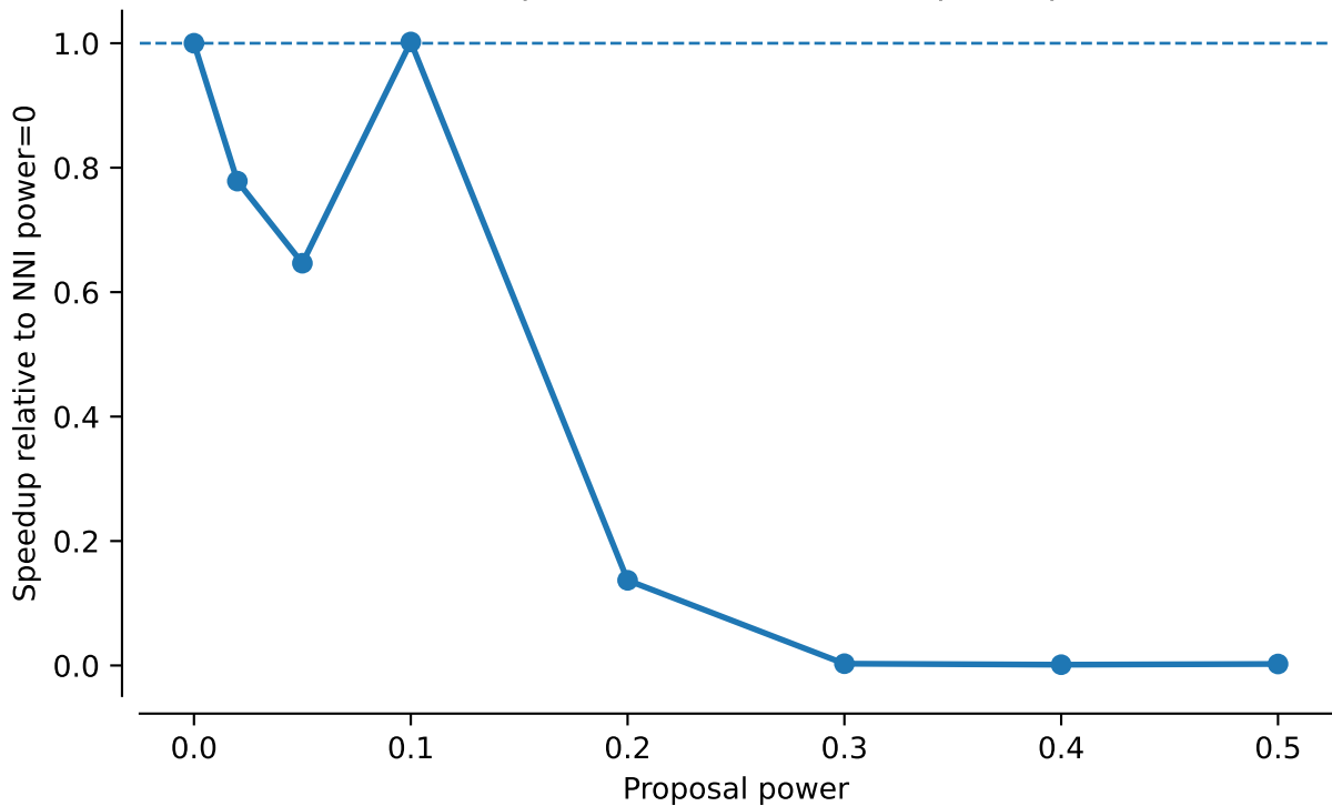
vert.atpase8.tw0: NNI tau95 speedup
