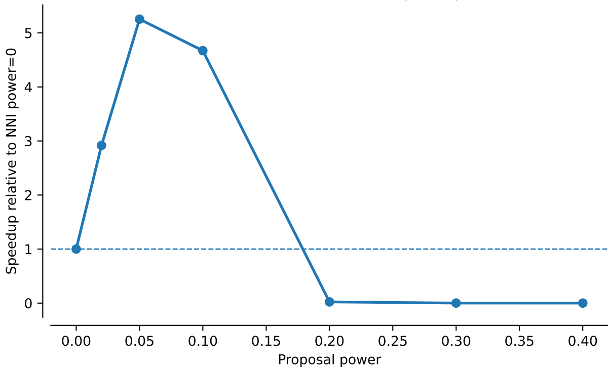
vert.nd4.tw0: NNI tau95 speedup
