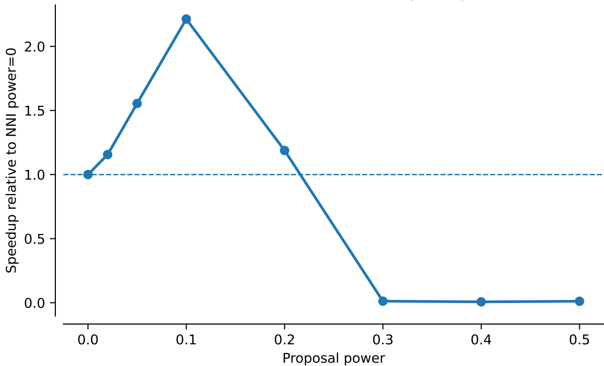
vert.nd4l.tw0: NNI tau95 speedup
