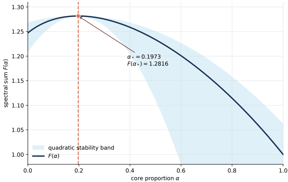
图 5.3: 平衡六分块模型的目标函数 F(\alpha) 及其二次稳定性带。虚线标出唯一最优比例 \alpha_* ; 阴影区域由定理 5.26 的两个二次界确定。
