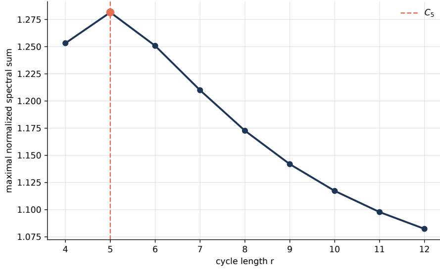
图 5.2: 平衡核心-环外围模型的最优归一化谱和。图中数值点由第八章的可复现脚本独立计算; theorem 5.7 已严格证明 r = 5 是唯一最大点。
