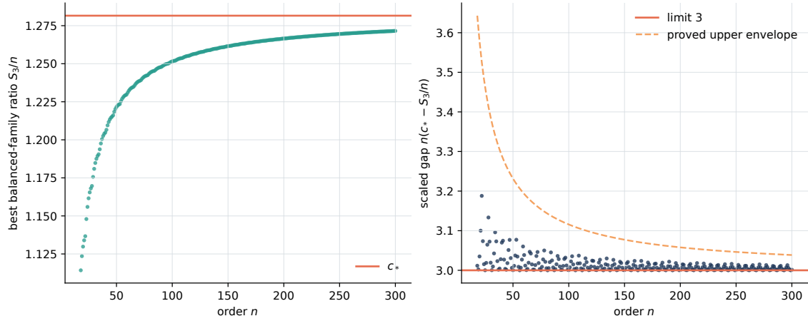
图 8.1: 平衡构造的有限阶收敛证据。左图给出最优平衡族比值 S_3(H_{a,b})/n 向 c_* 的趋近；右图给出缩放误差 n(c_* - S_3/n) 以及 corollary 5.17 的显式包络。
