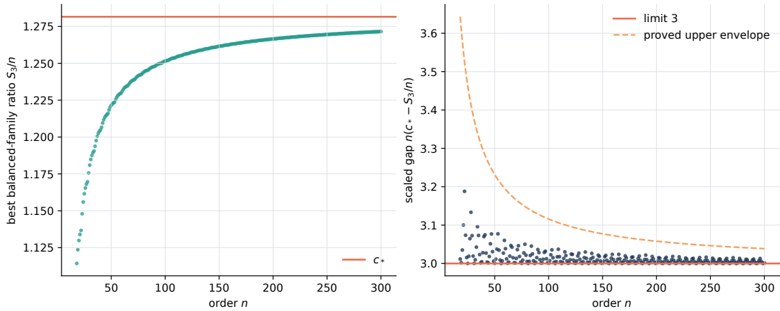
图 8.1: 平衡构造的有限阶收敛证据。左图给出最优平衡族比值 S_3(H_{a,b})/n 向 c_* 的趋近；右图给出缩放误差 n(c_* - S_3/n) 以及推论 5.44 的显式包络。
