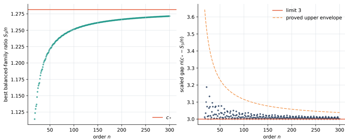
图 8.1: 平衡构造的有限阶收敛证据。左图给出最优平衡族比值 S_3(H_{a,b})/n 向 c_* 的趋近；右图给出缩放误差 n(c_* - S_3/n) 以及推论 5.51 的显式包络。
