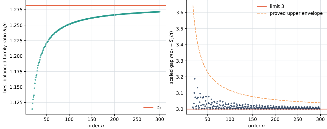
图 8.1: 平衡构造的有限阶收敛证据。左图给出最优平衡族比值 S_3(H_{a,b})/n 向 c_* 的趋近；右图给出缩放误差 n(c_* - S_3/n) 以及推论 5.47 的显式包络。
