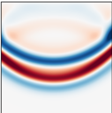
Truth · t=200
