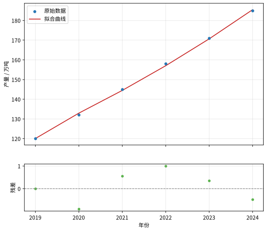
图 1: GM(1,1) 拟合效果与残差分布
