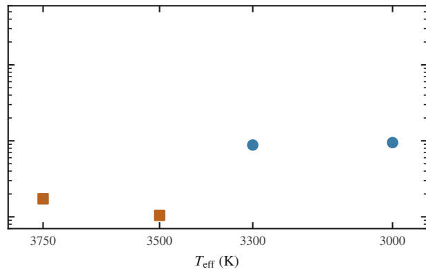
(d) retained M-giant atmospheres
