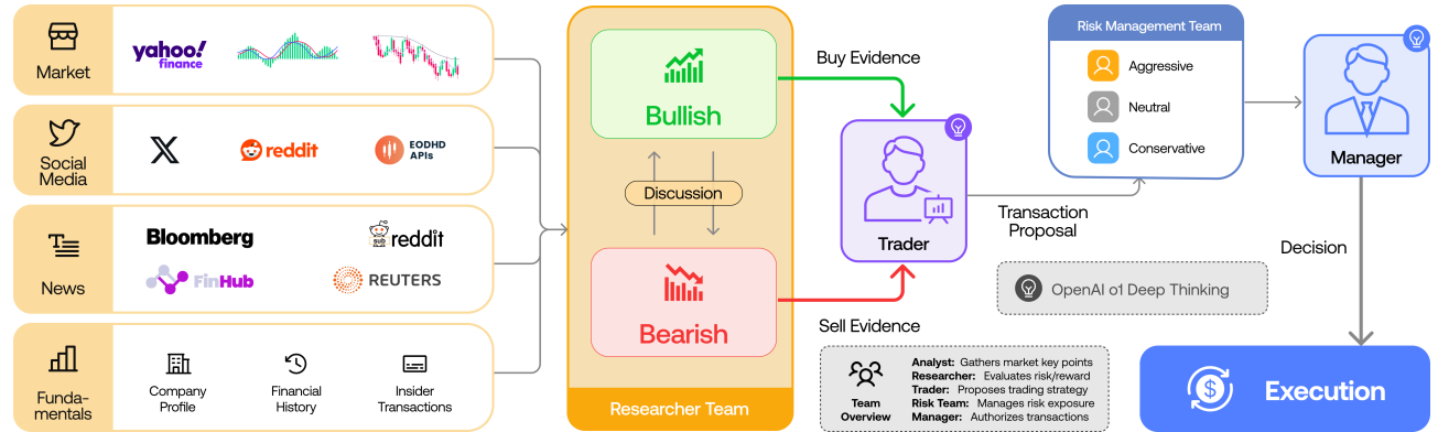
Fig. 1: TradingAgents 框架总览。一、分析师团队：四位分析师同时收集相关的市场信息。二、研究团队：团队讨论并评估收集到的数据。三、交易员：交易员根据研究人员的分析做出交易决策。四、风险管理团队：风险管理人员根据当前市场状况评估该决策，以降低风险。五、基金经理：基金经理批准并执行交易。
