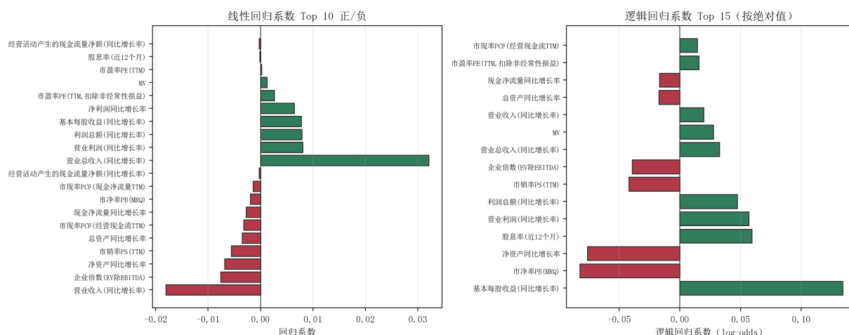
图4 线性回归与逻辑回归系数对比
