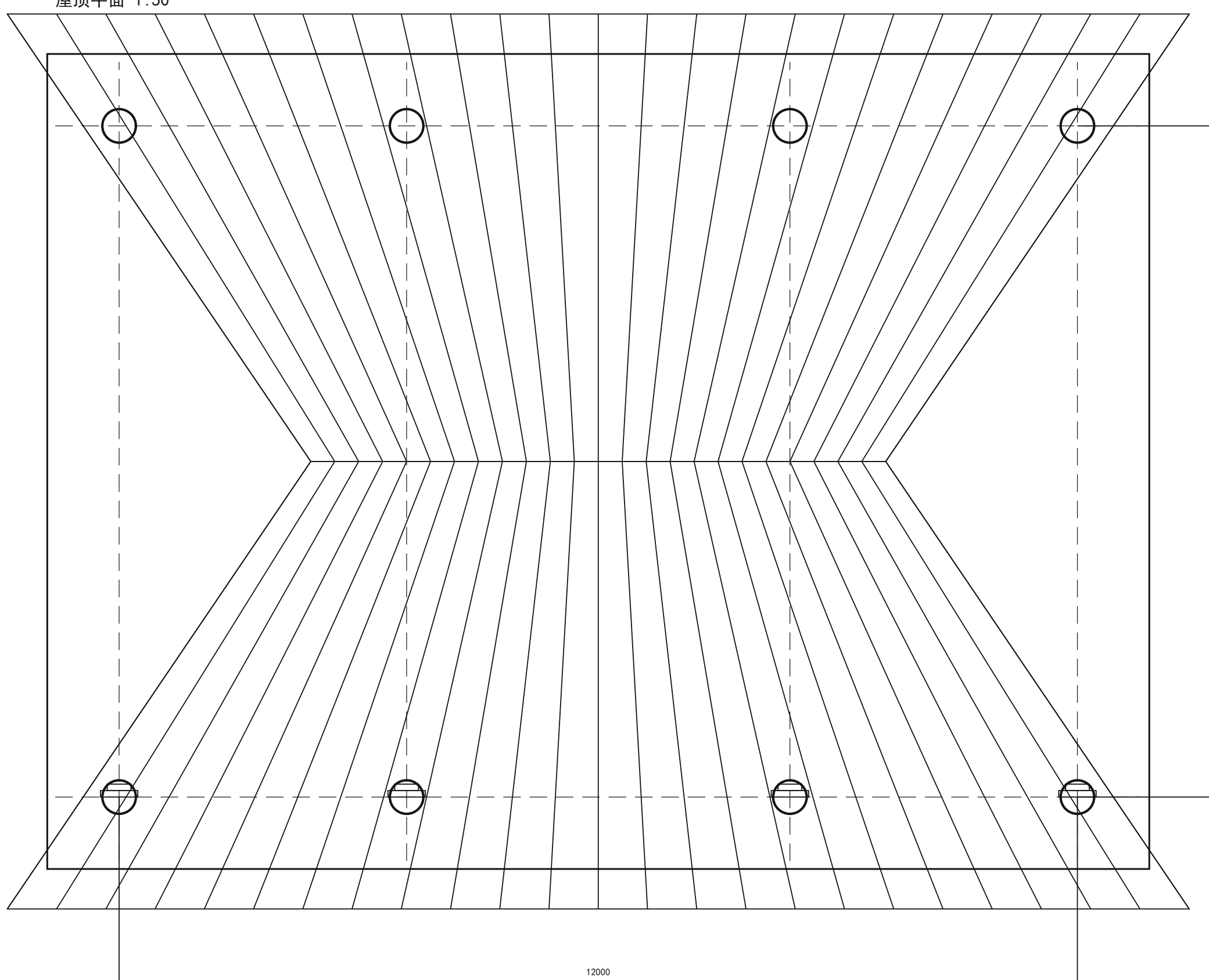
屋顶平面 1:50
