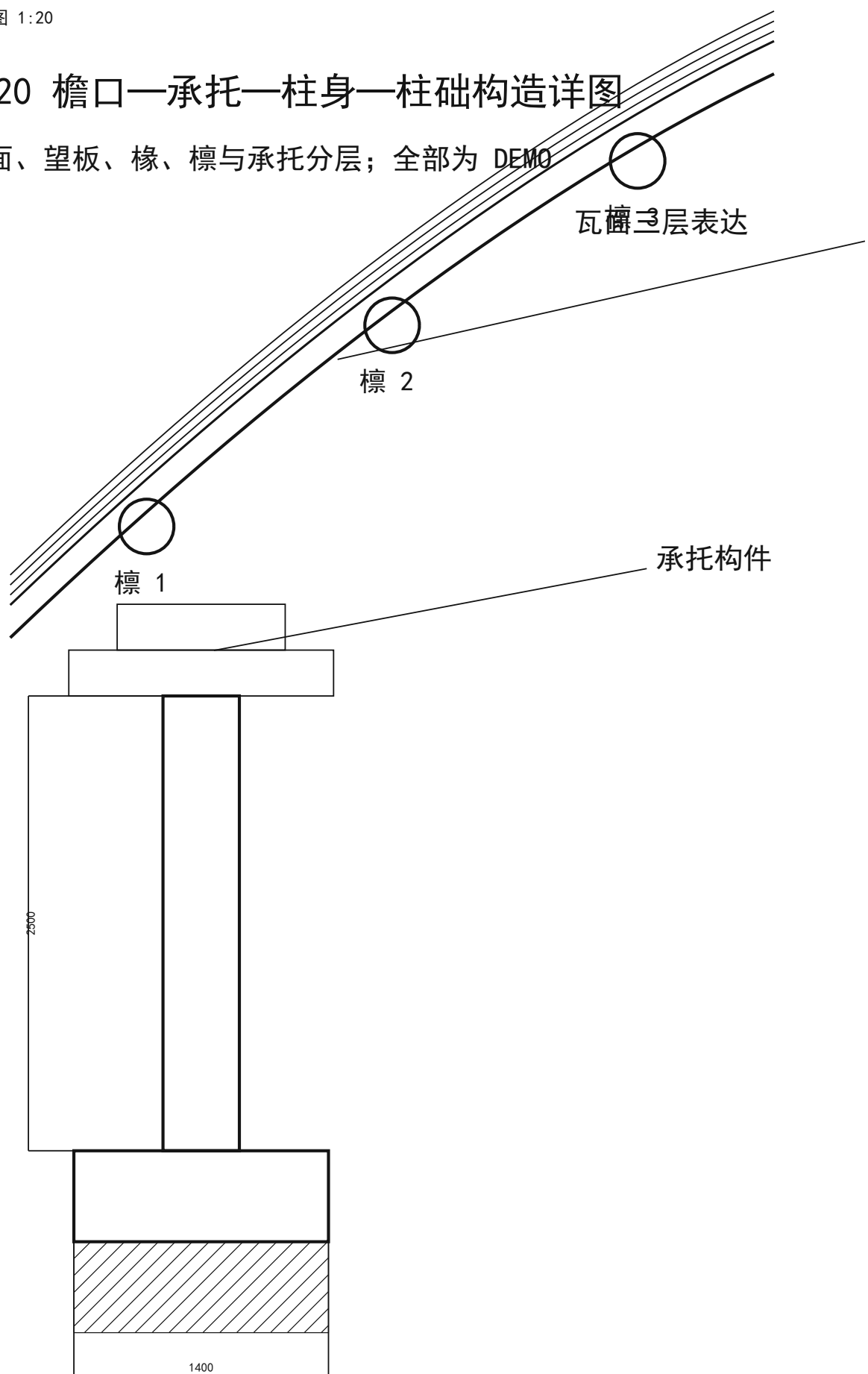
檐口构造详图 1:20
