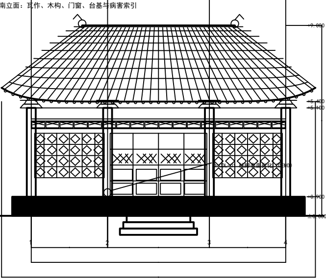
南立面 1:50
