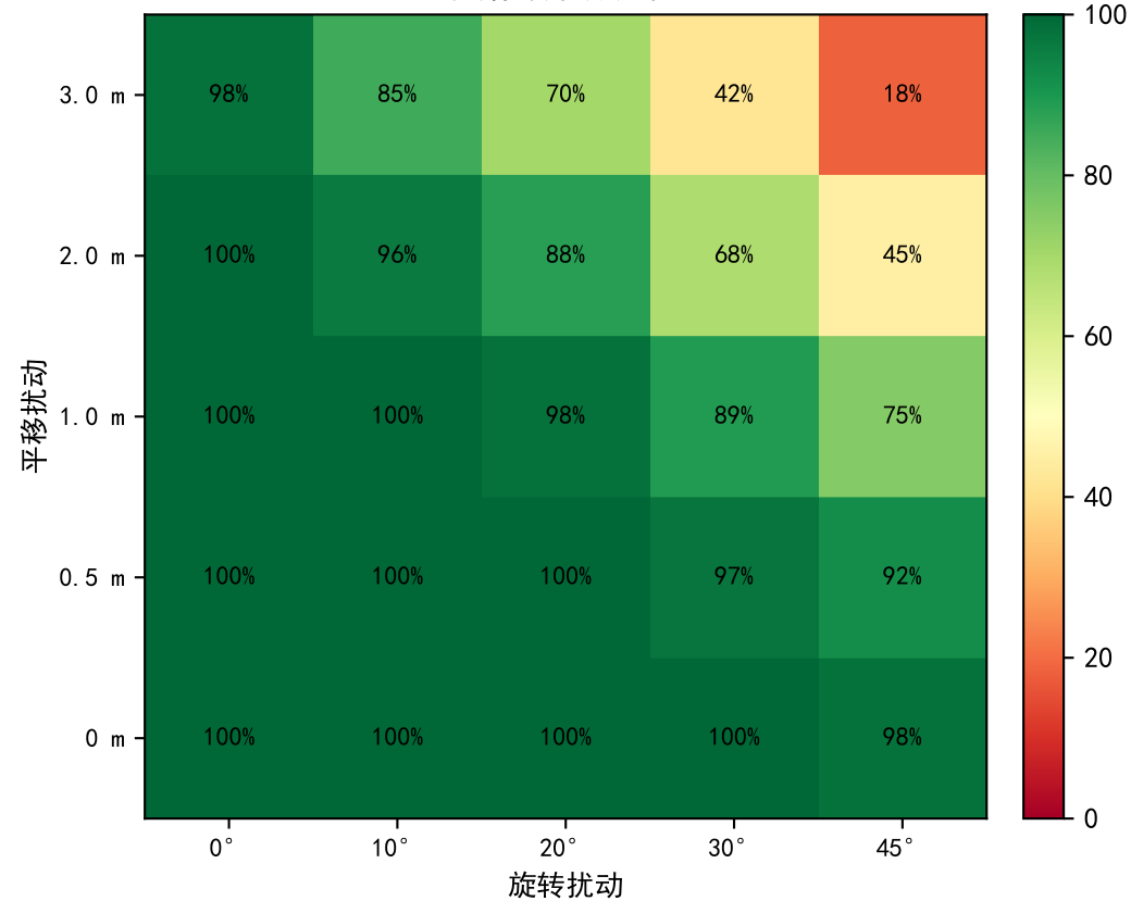
ICP 初始对齐成功率 (%)
