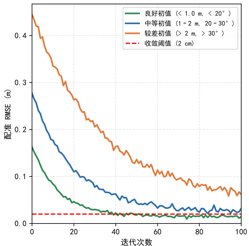
ICP 残差收敛曲线
