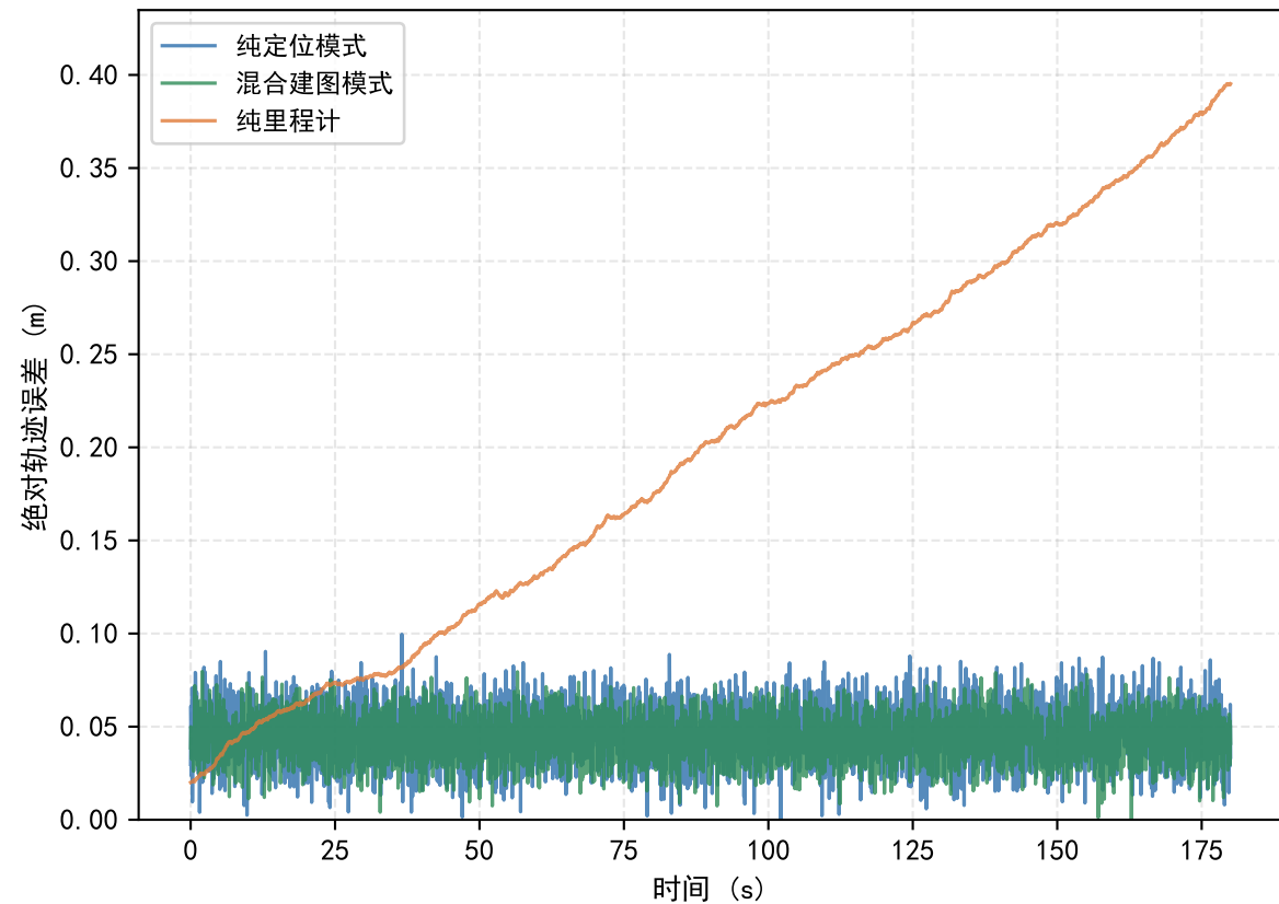
迷宫场景 APE 时间序列
