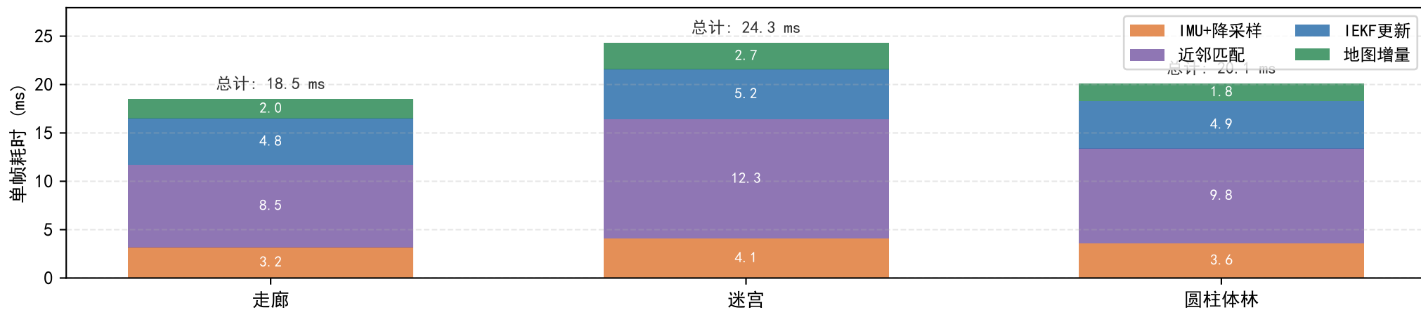
各模块平均耗时分解
