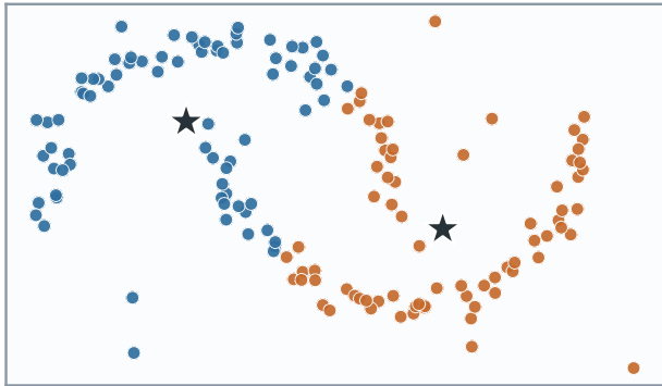
(a) K-Means (非凸数据被错误切分)
