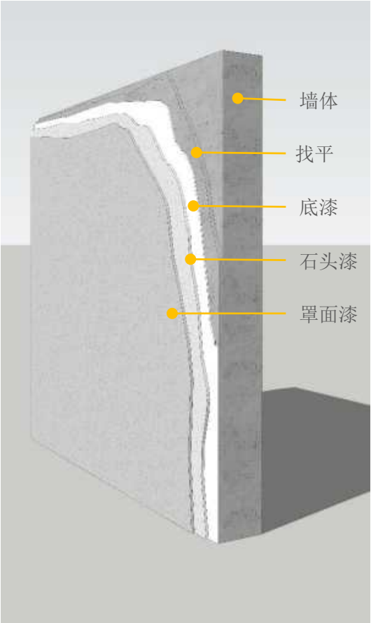
次要外饰面喷涂真石漆
