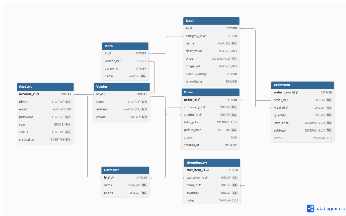
圖 1 ER Diagram 圖
