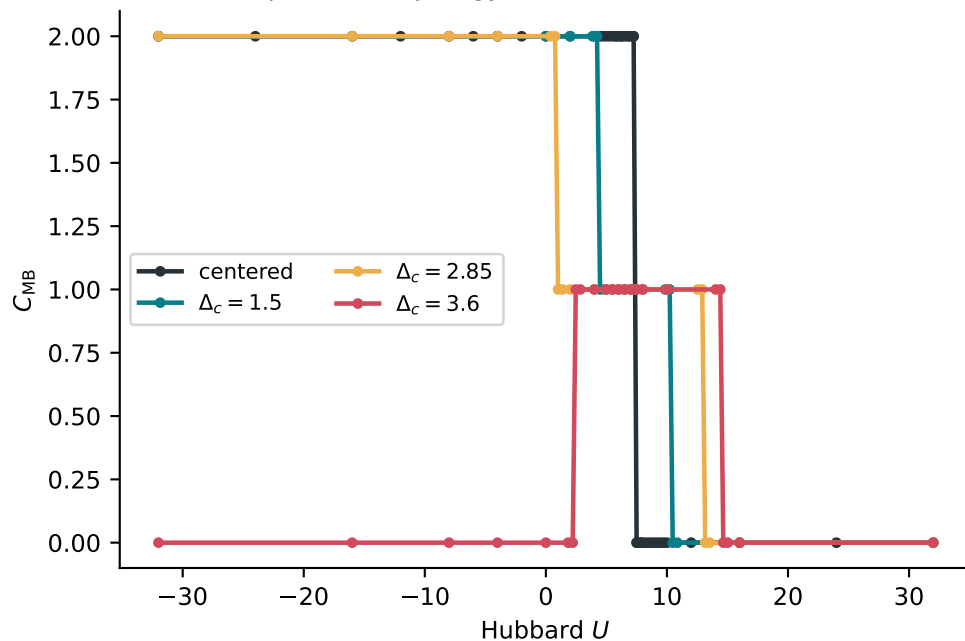
(d) Twist-averaged topological efficiency
