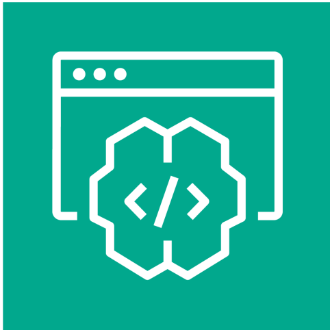
CodeWhisperer
