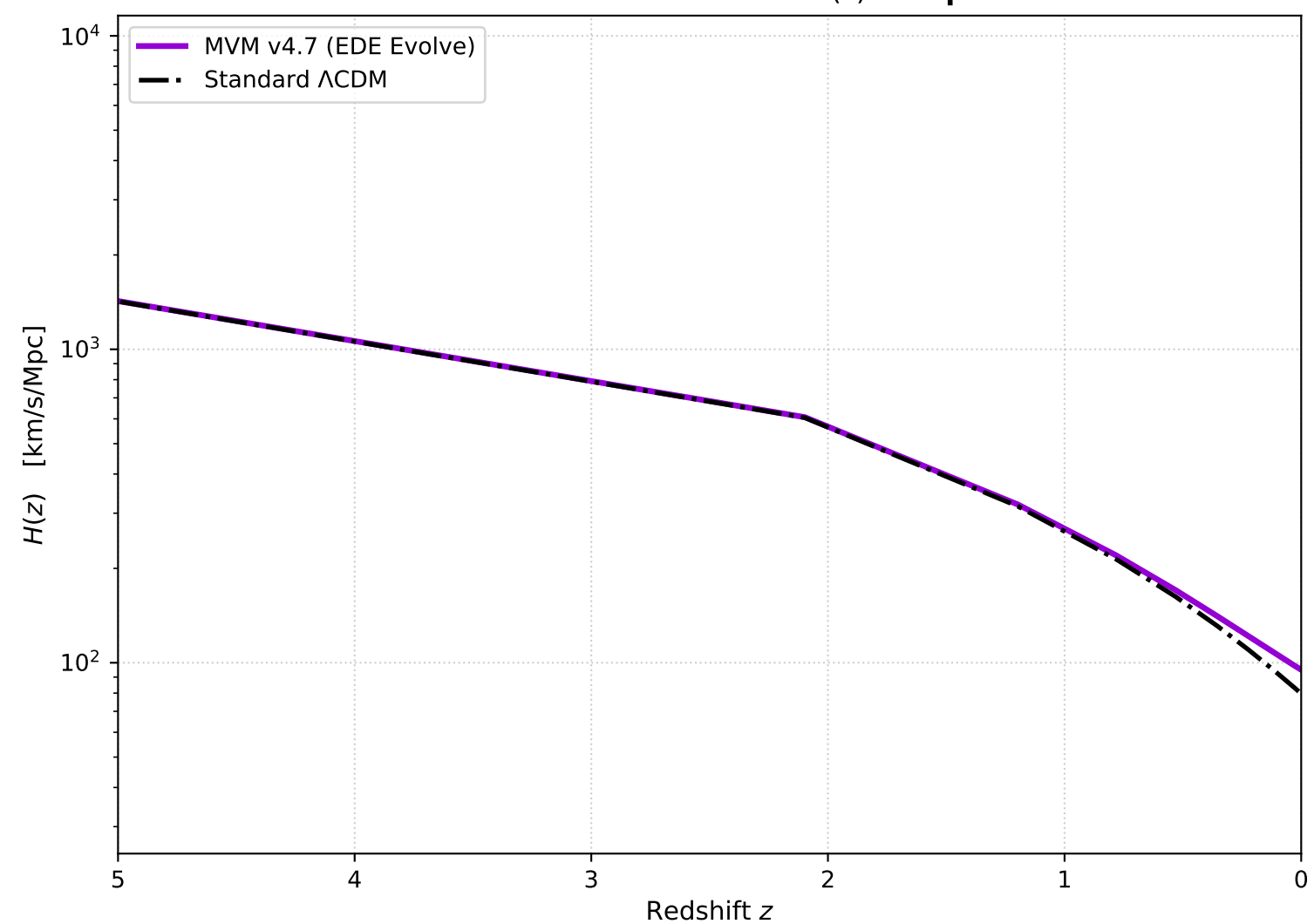
Hubble Parameter Evolution H(z) Comparison
