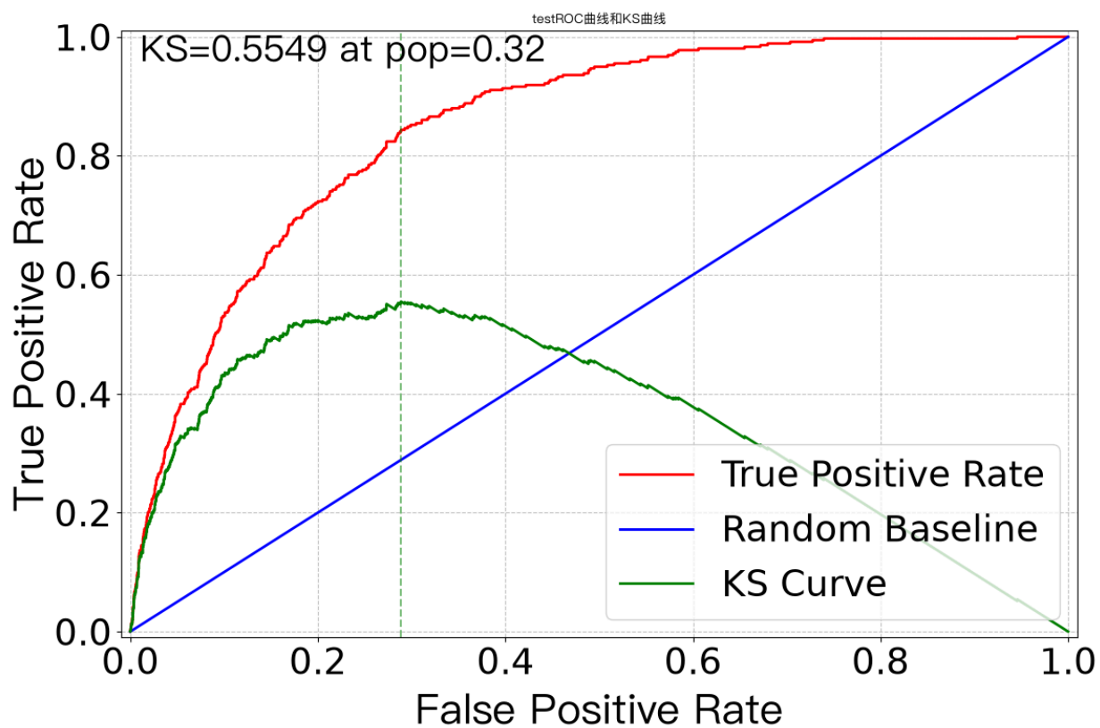
图10 平台验证-开发验证集（2023）：AUC 0.850 / KS 0.555
