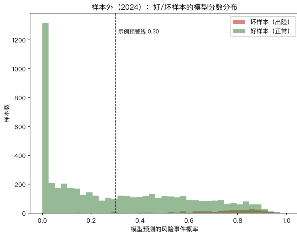
图3 样本外好坏样本的分数分布：出险公司集中在高概率区，正常公司集中在低概率区——分离清晰
