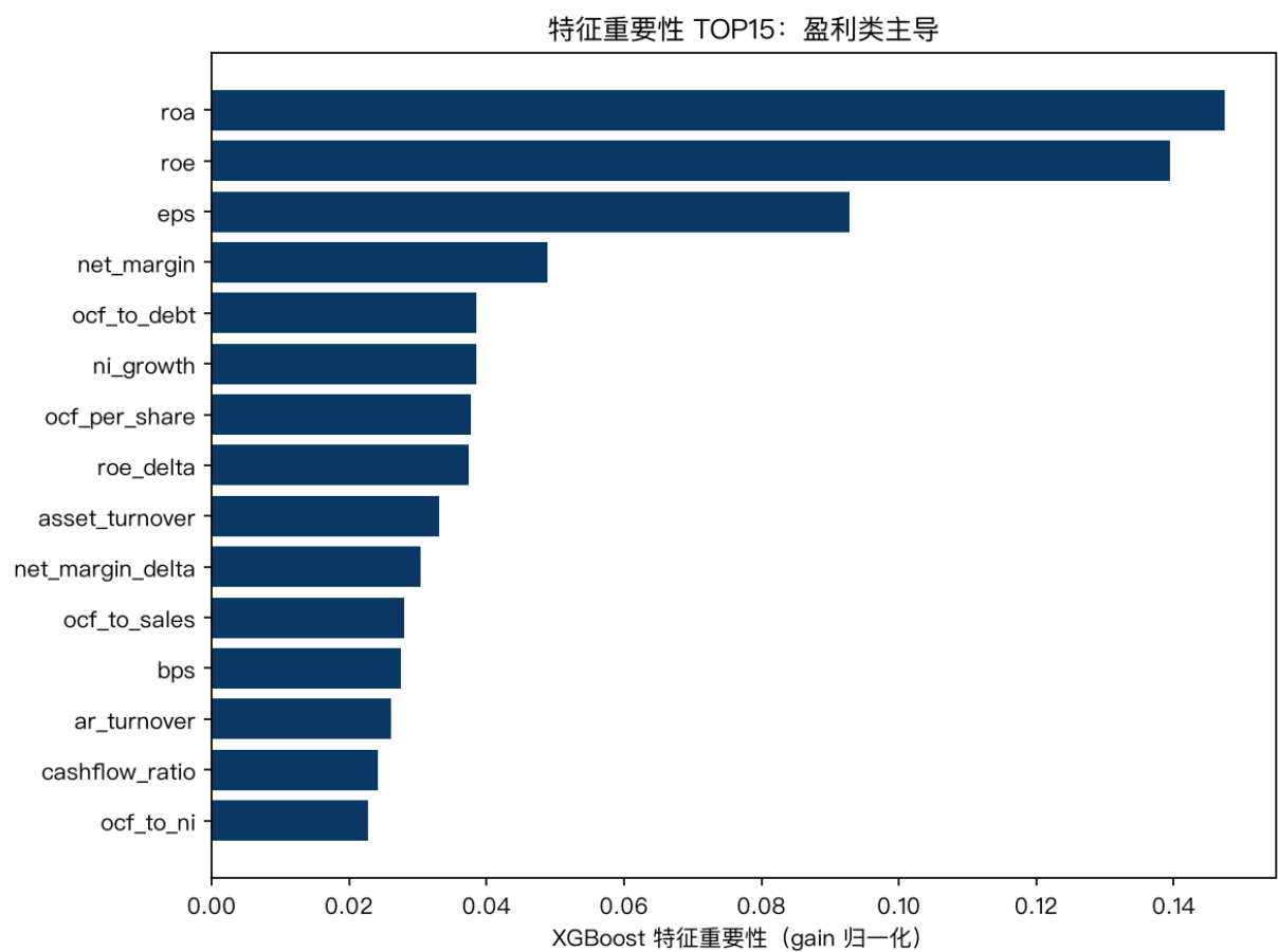
图4 特征重要性TOP15：ROE/EPS/ROA/净利率等盈利类霸榜——模型核心依赖"盈利质量"，与信用分析理论一致
