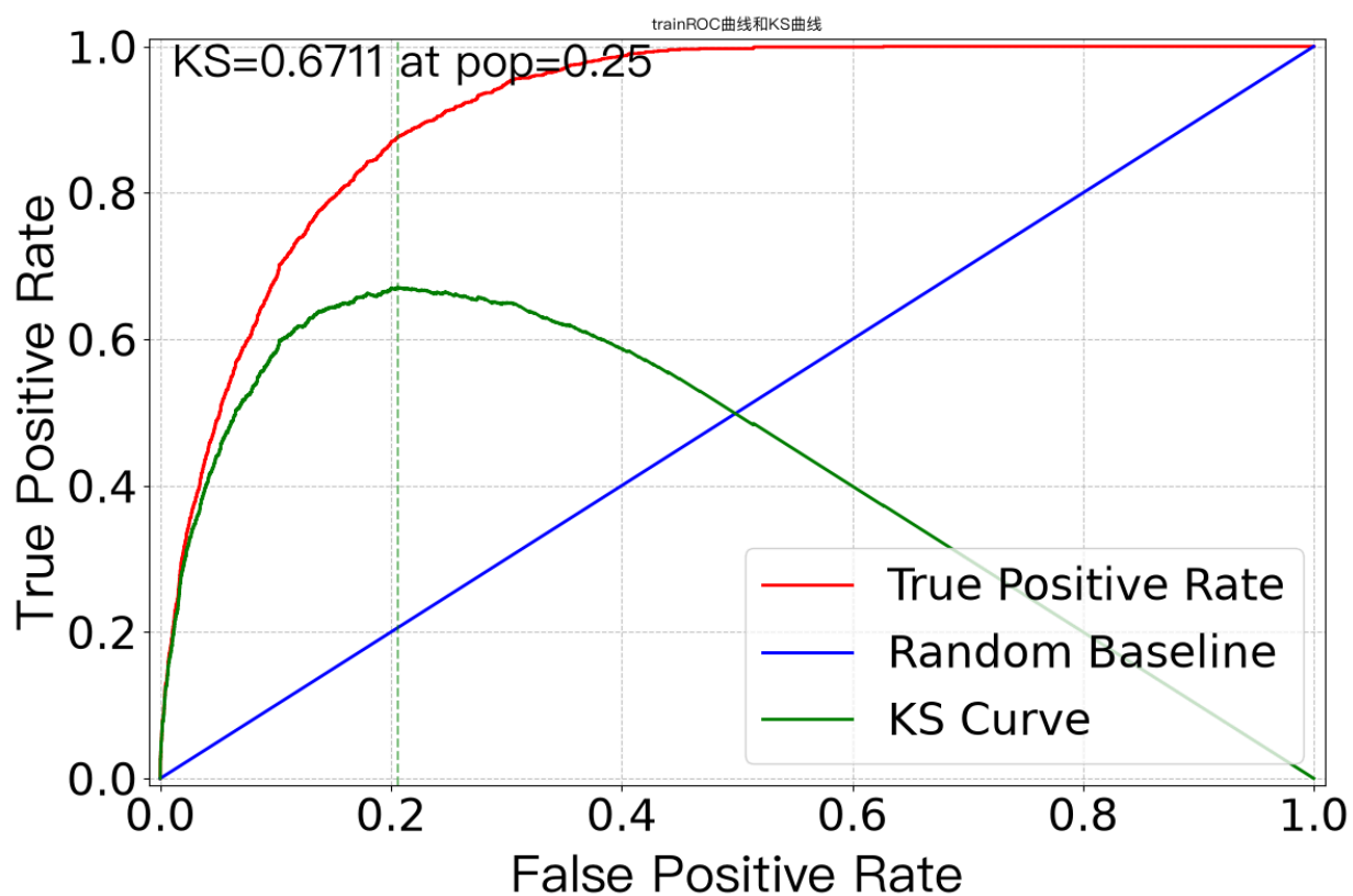
图9 平台验证-训练集（2019-2022）：AUC 0.912 / KS 0.671
