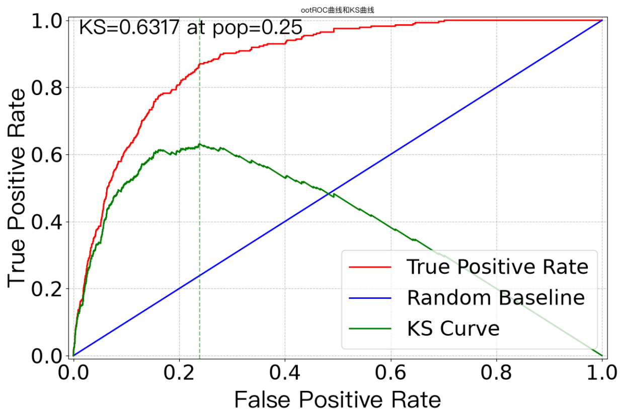
图11 平台验证-样本外（2024+2025）：AUC 0.882 / KS 0.632——平台独立内核计算结果，与本地评估互相印证
