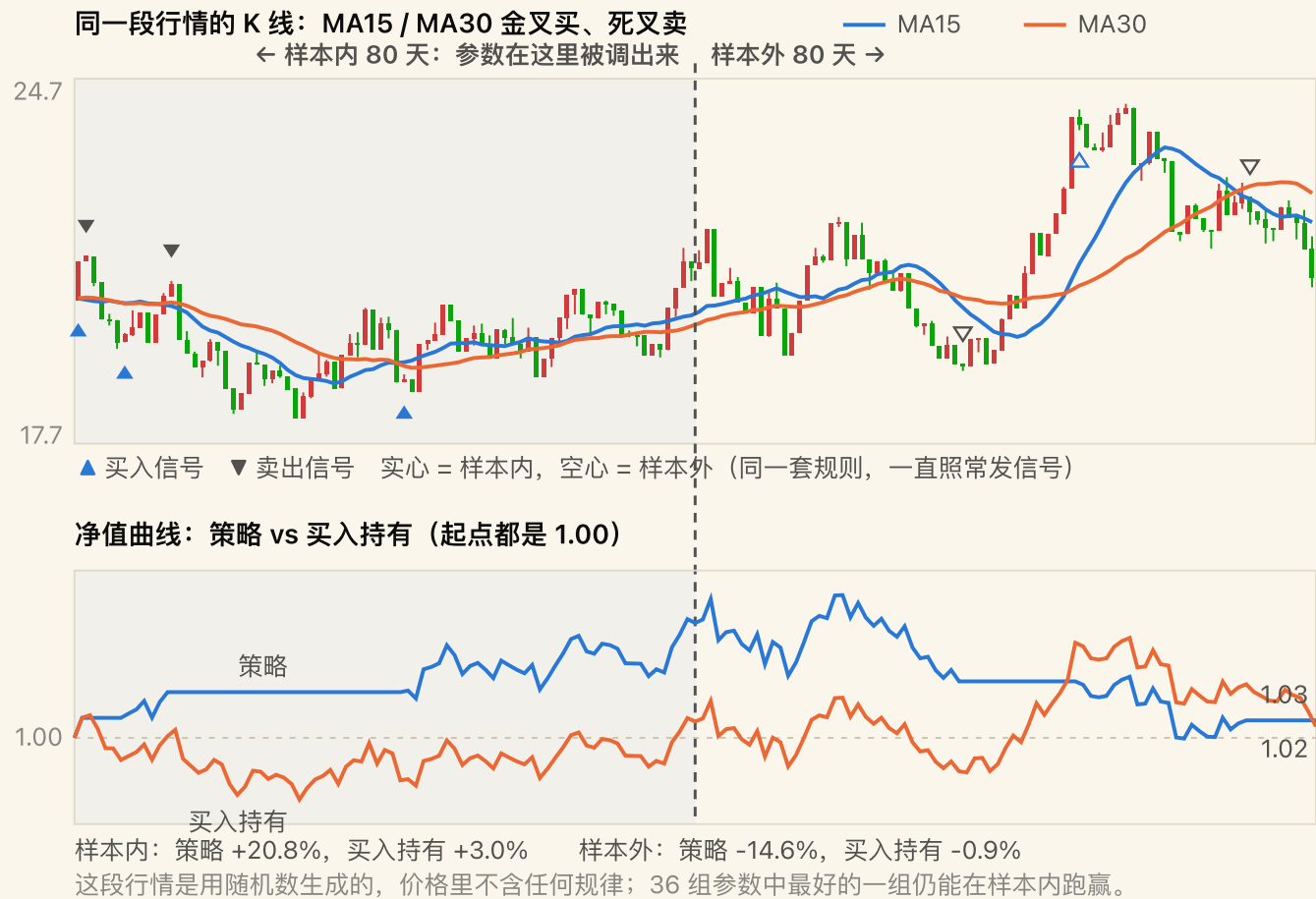
图 4-3 · 一次教科书式的过拟合
