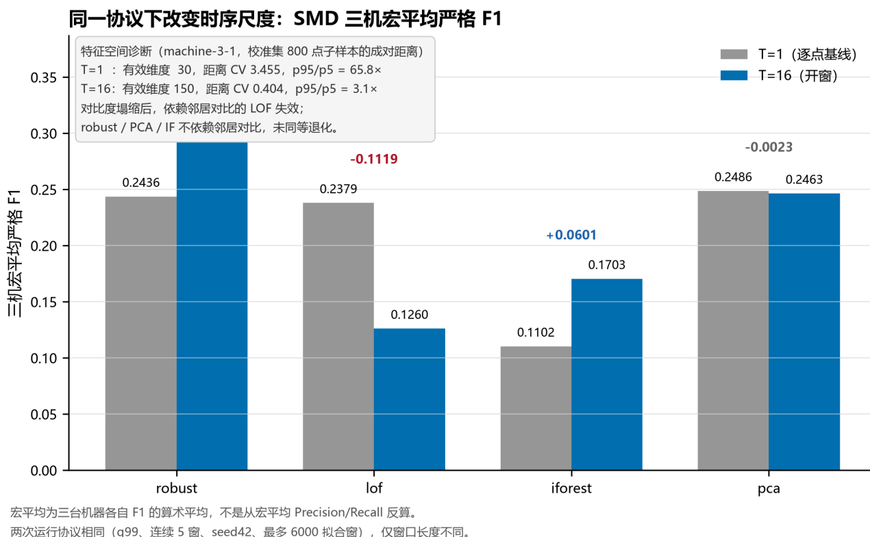
图 5 四方法 × 两尺度的宏平均严格 F1 对比, 图中诊断框给出特征空间的成对距离对比度。
