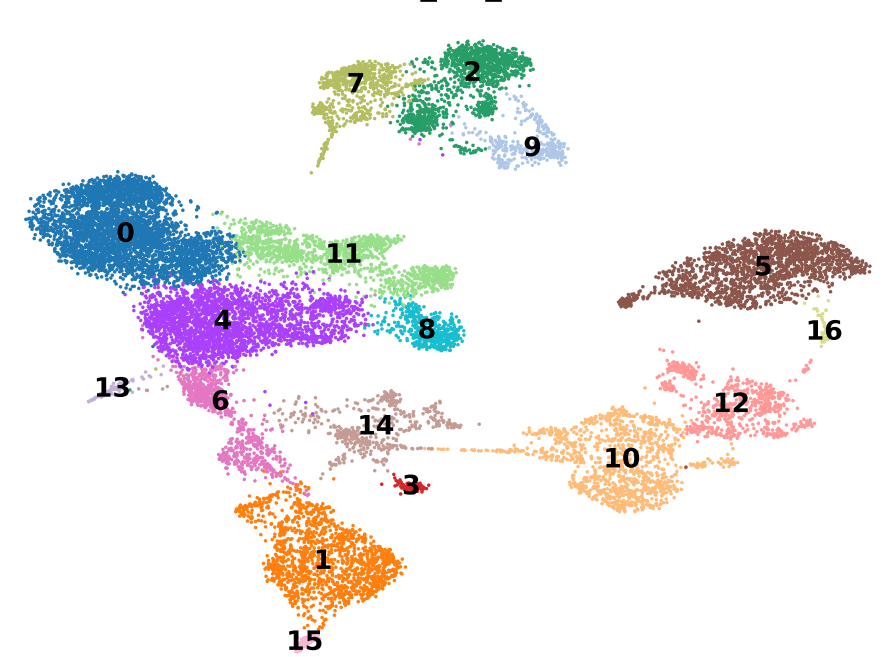
leiden_res_0.50
