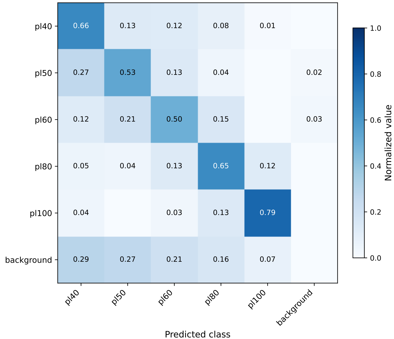
ECAFA-YOLO+KD
