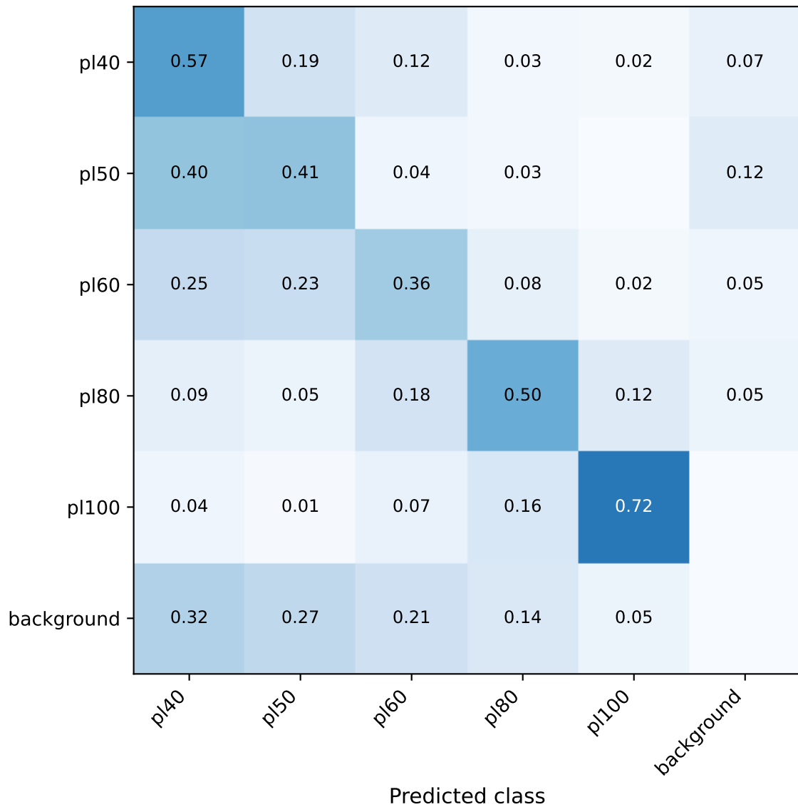
YOLOv11
