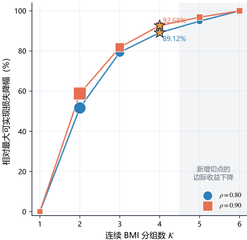
(a) 分组数—决策损失帕累托前沿
