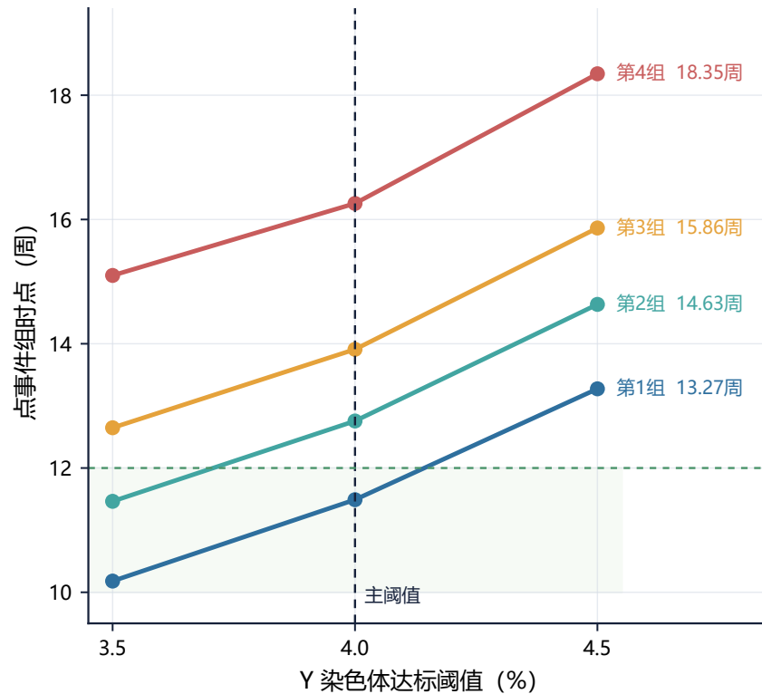
(b) 阈值变化的组时点斜率图
