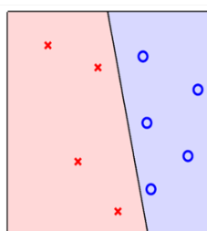
线性可分
