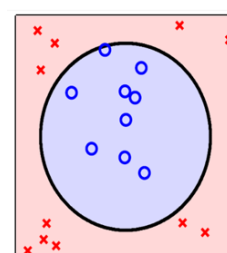
线性不可分
