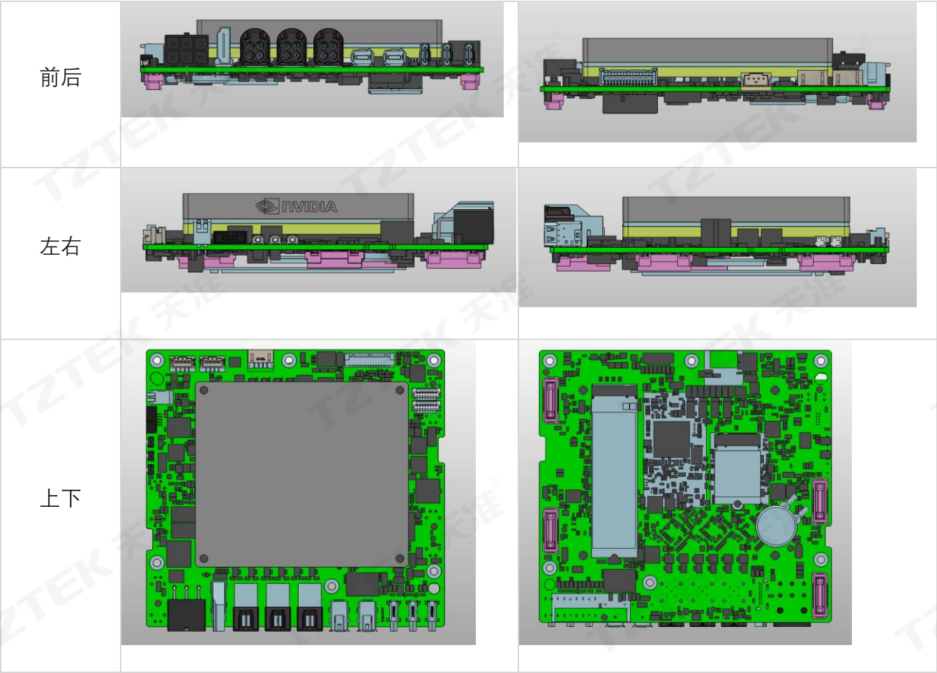
全配版本产品实物图
